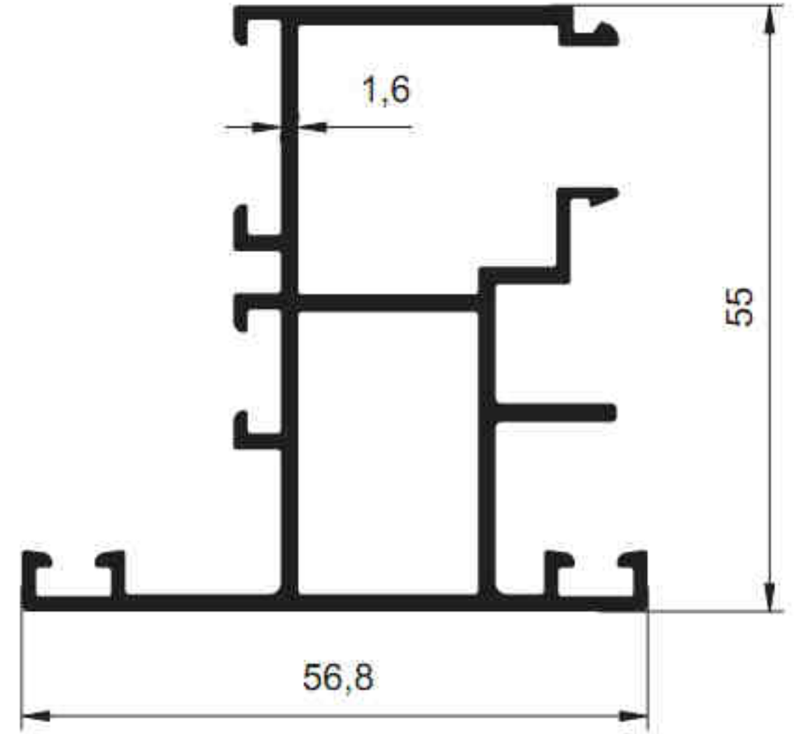
3145 - 1.108 kg/m
