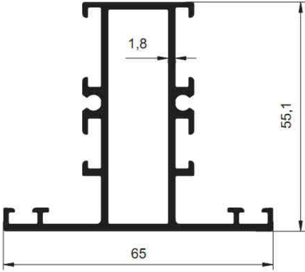
3256 - 1.244 kg/m
