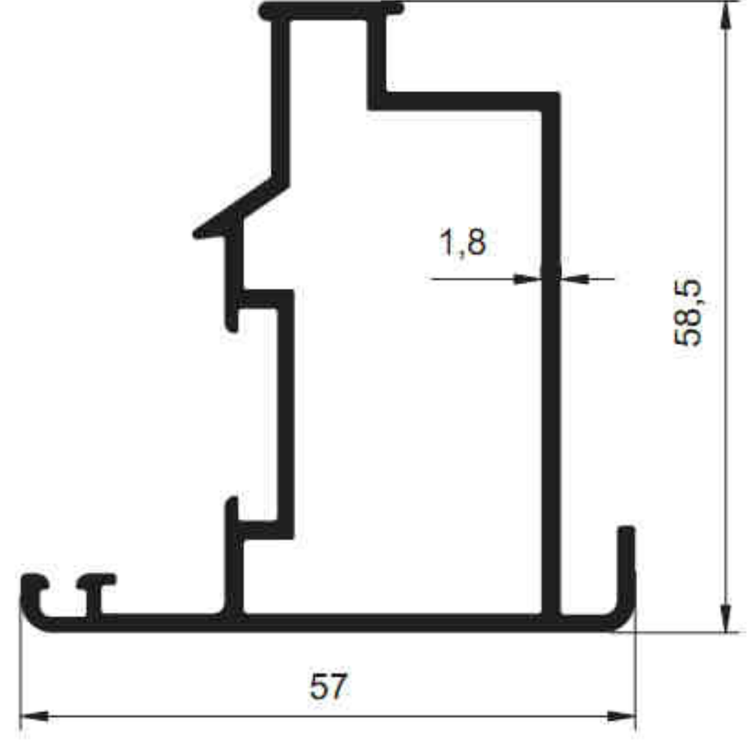
3341 - 1.093 kg/m
