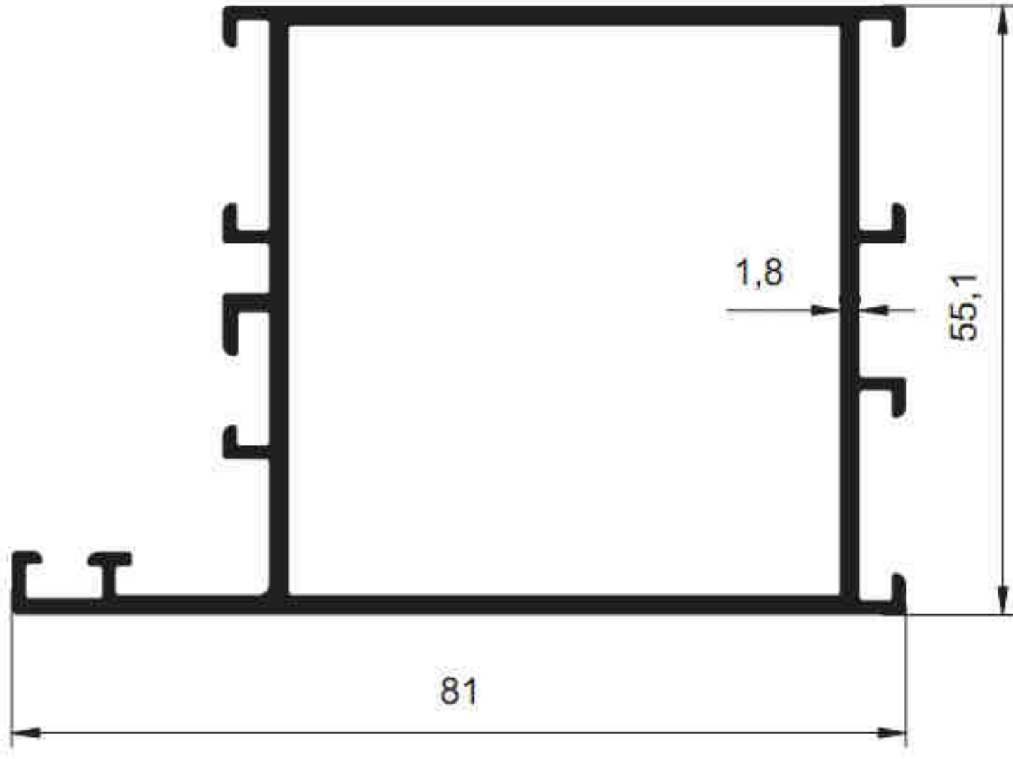
3340 - 1.357 kg/m
