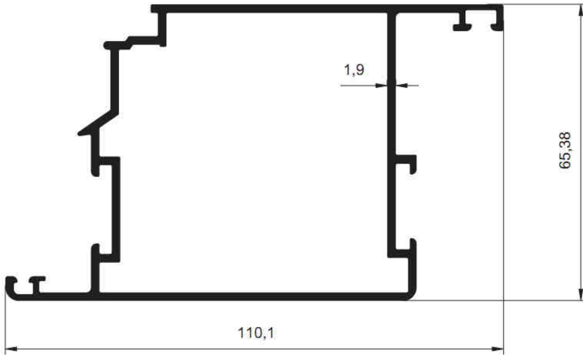
3144 - 1.788 kg/m
